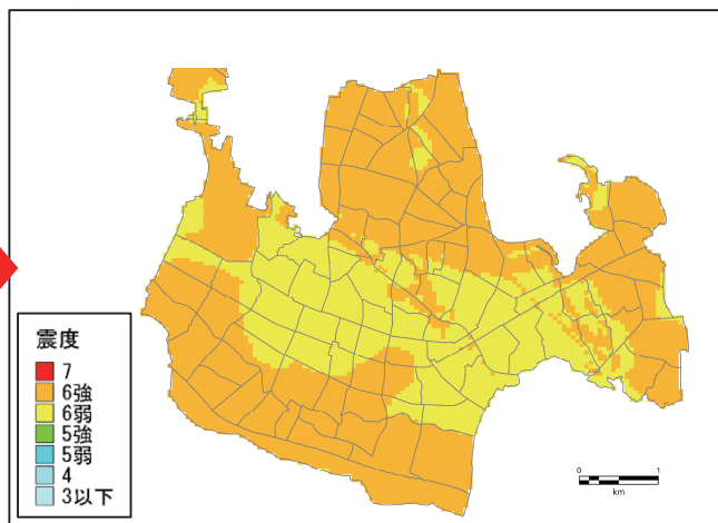
多摩東部直下地震（M7.3）令和5年想定
