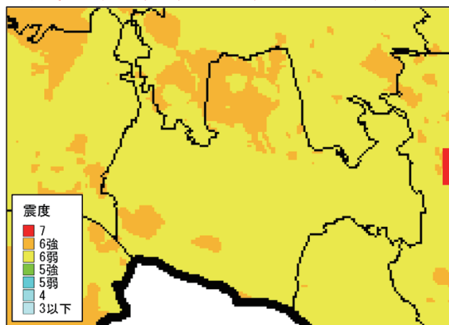
多摩直下地震（M7.3）平成24年想定
