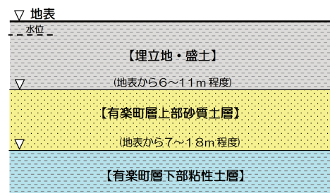
図 2-5 臨海部の埋立地盤の地層構成の例
