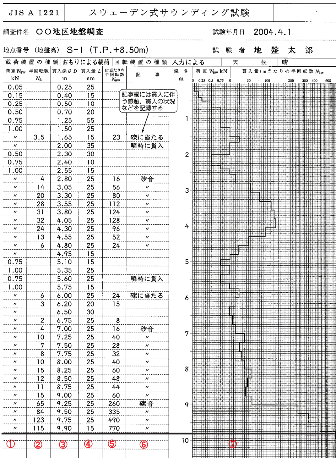
図 6-2 スクリーウエイト貫入試験の調査結果の例
