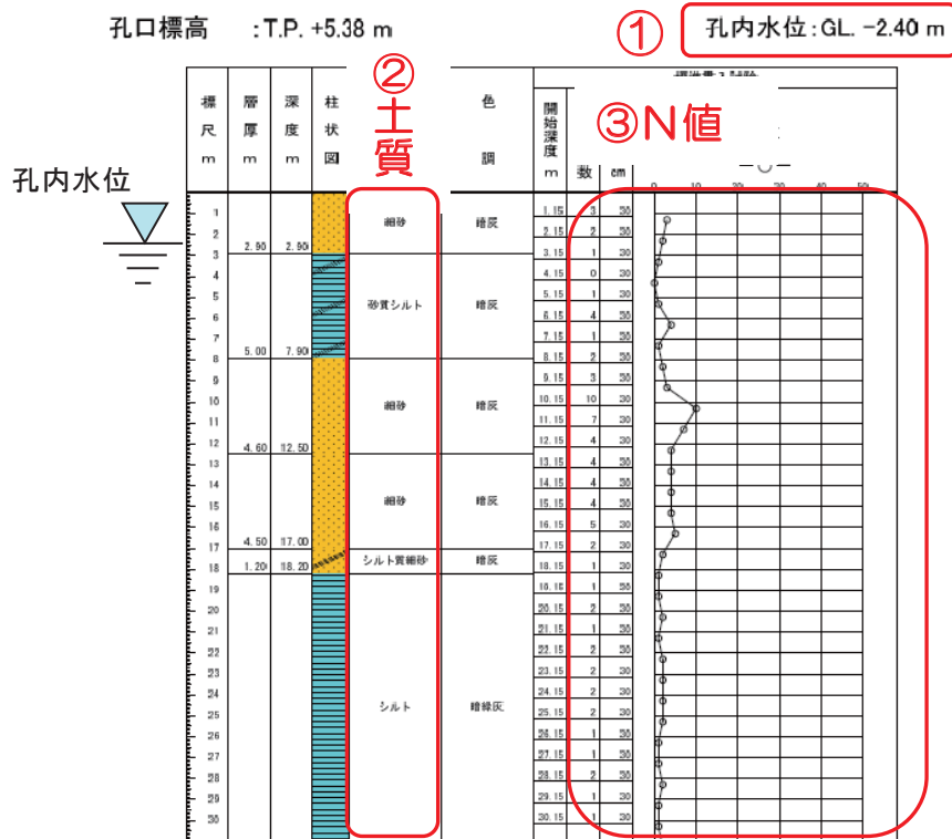
図 5-6 ボーリング柱状図の表記例
