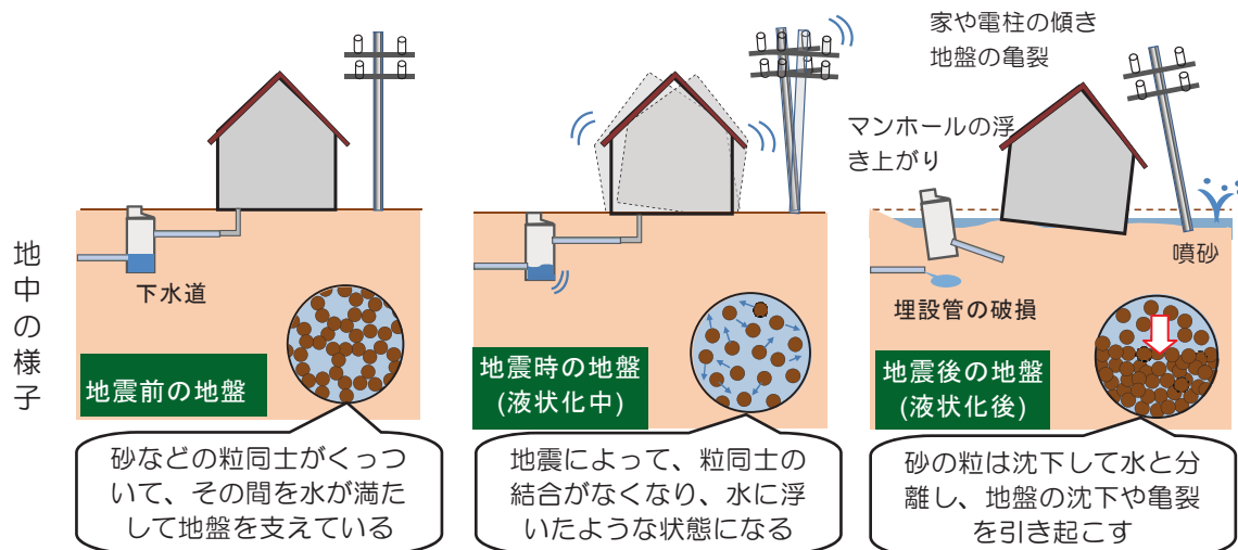
図 2-2 液状化発生仕組み
