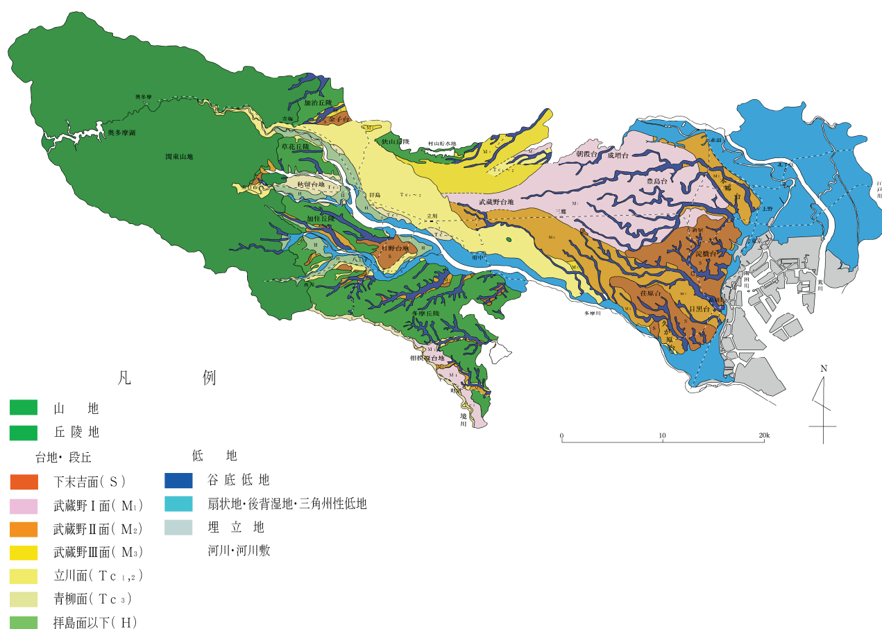
図 2-3 東京の地形区分図
