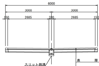
区画道路1号・3号 標準断面図
