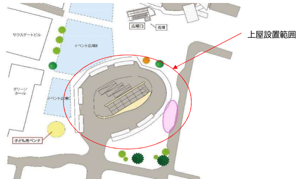
調布駅北側ロータリー上屋(整備済)
