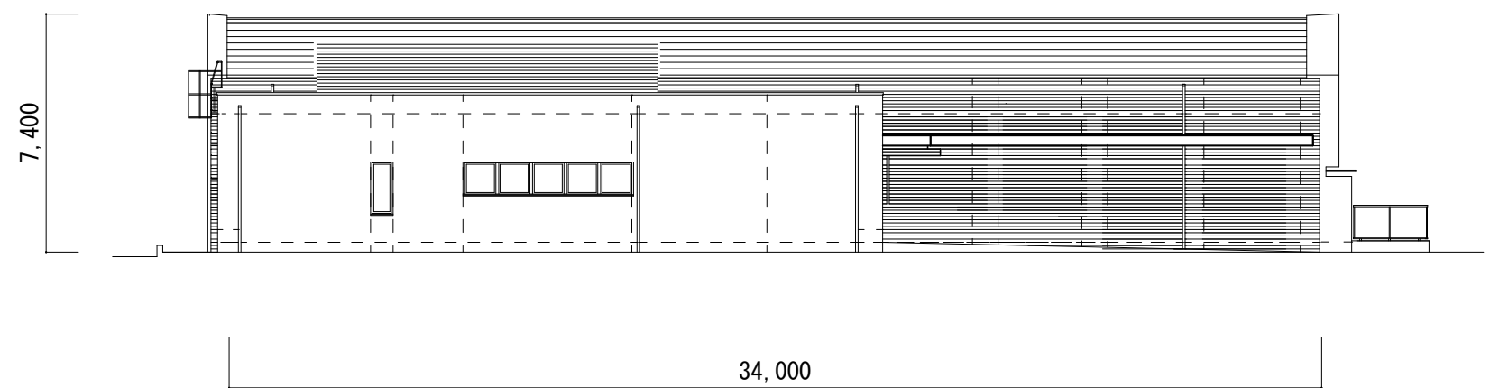
北東立面图
