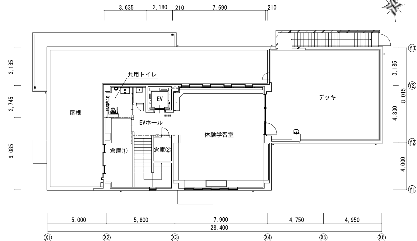
2 階平面図
