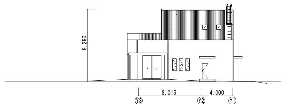
西立面図
