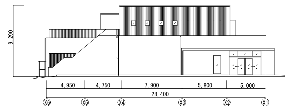
北立面図
