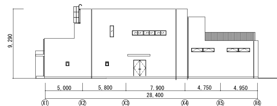
南立面図
