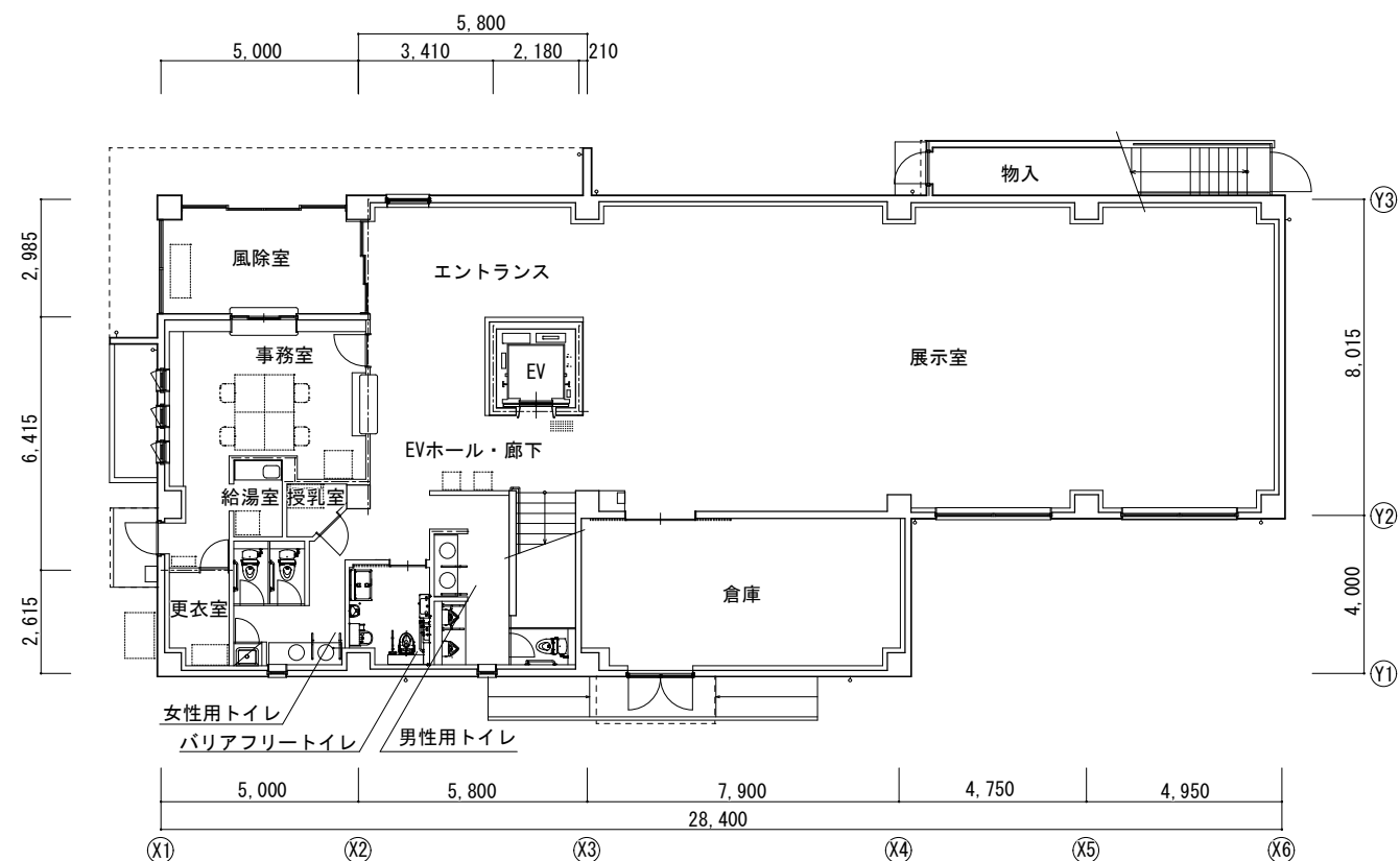
1 階平面図
