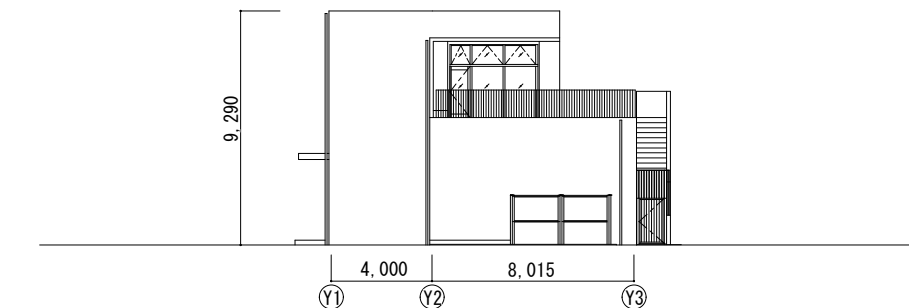
東立面図
