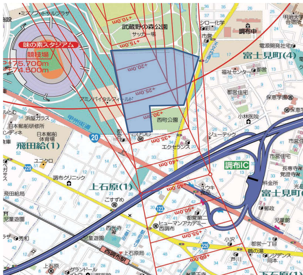
図表5 調布飛行場 制限表面図
