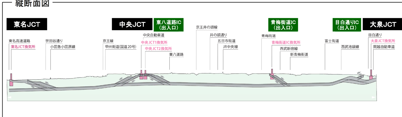
縦断面図
