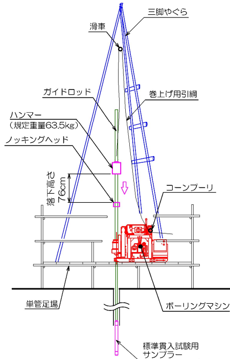
装置の概要図
