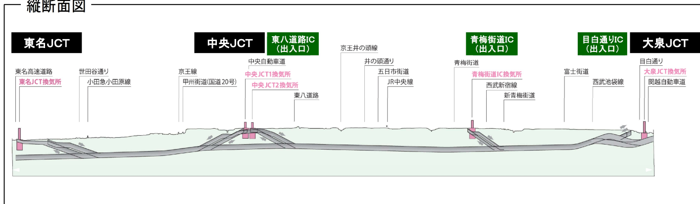
縦断面図
