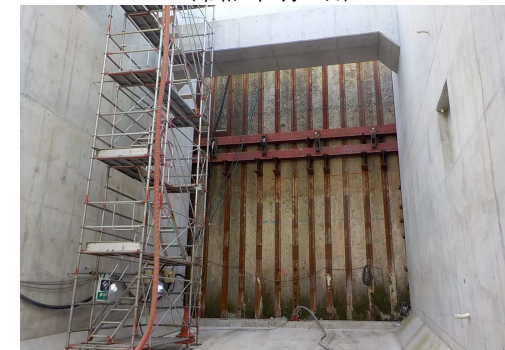
中央JCT北側開削トンネル施工状況 (令和5年2月1日)
